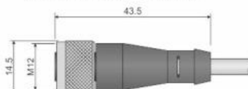
Connettore femmina M12 - versione dritta M12 female connector - straight type
