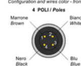
Configurazione e colori - vista lato frontale Configuration and wires color - front view
