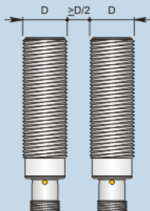
Montaggio affiancato
