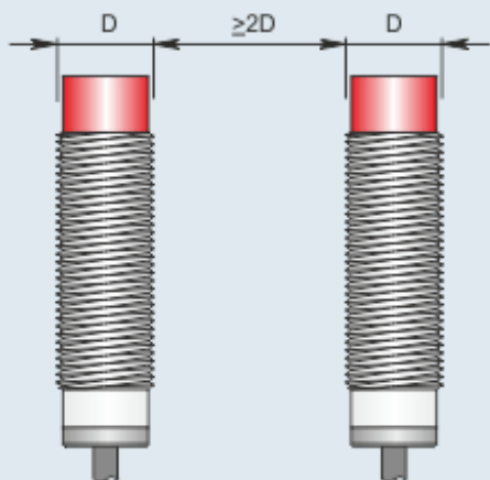
Montaggio affiancato
