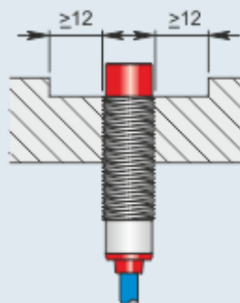
Montaggio sporgente
