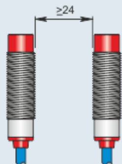
Montaggio affiancato
