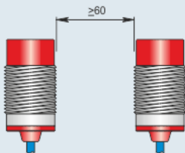
Montaggio affiancato
