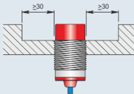
Montaggio sporgente
