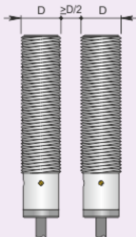
Montaggio affiancato
