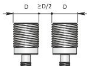
Montaggio affiancato
