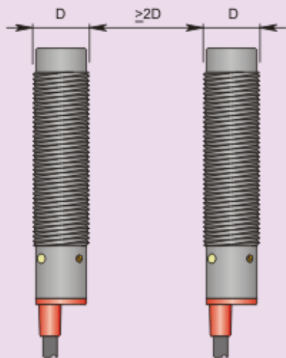
Montaggio affiancato
