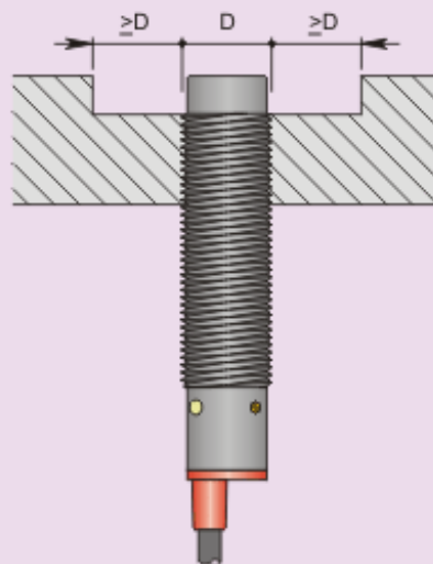
Montaggio sporgente
