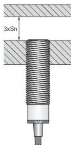
Montaggio a filo
