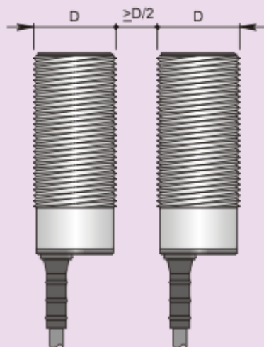
Montaggio affiancato
