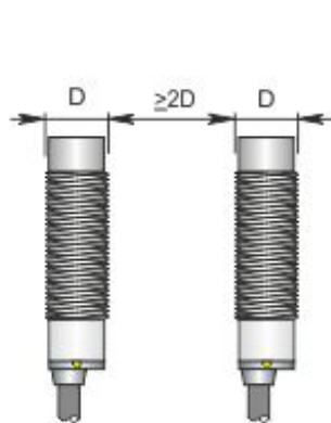
Montaggio affiancato
