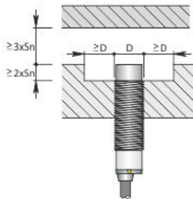
Montaggio spogente
