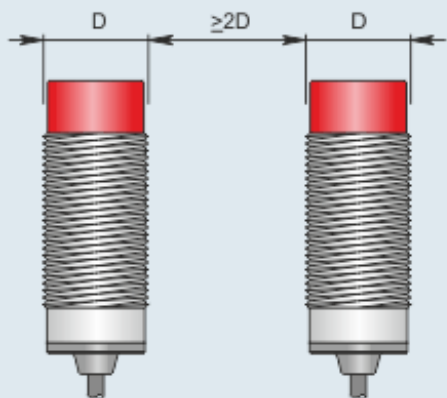
Montaggio affiancato
