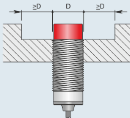
Montaggio sporgente
