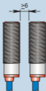
Montaggio affiancato
