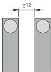
Montaggio affiancato
