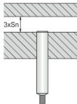
Montaggio a filo
