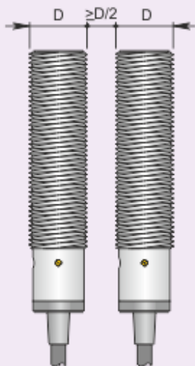
Montaggio affiancato
