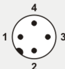
VISTA DEL CONNETTORE MASCHIO
