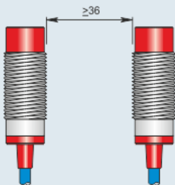
Montaggio affiancato
