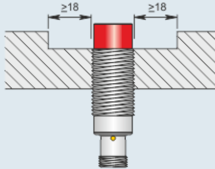
Montaggio sporgente
