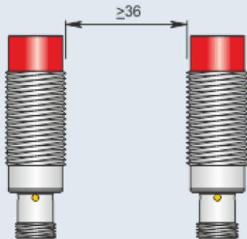
Montaggio affiancato
