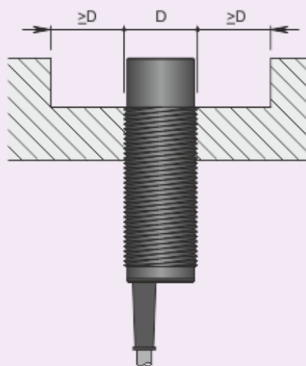
Montaggio sporgente
