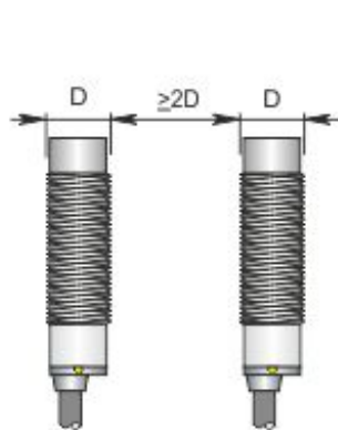
Montaggio affiancato
