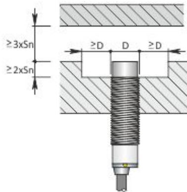
Montaggio spogente
