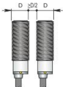
Montaggio affiancato
