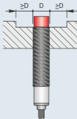
Montaggio sporgente
