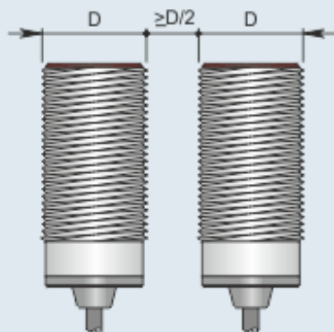
Montaggio affiancato
