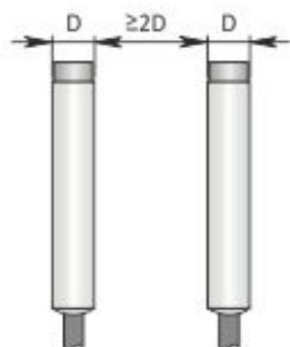
Montaggio affiancato
