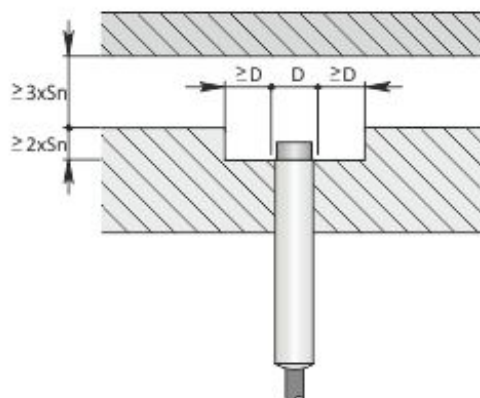
Montaggio spogente
