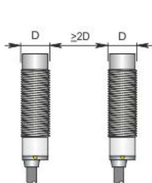
Montaggio affiancato
