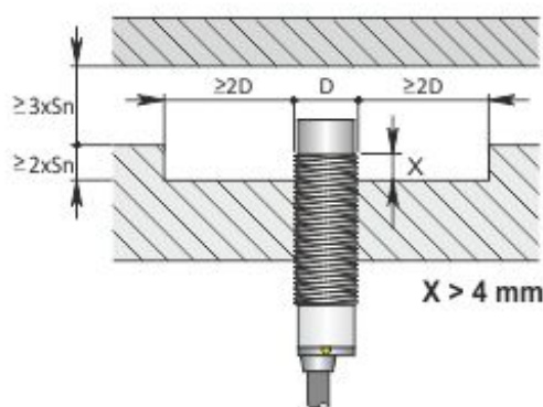
Montaggio spogente
