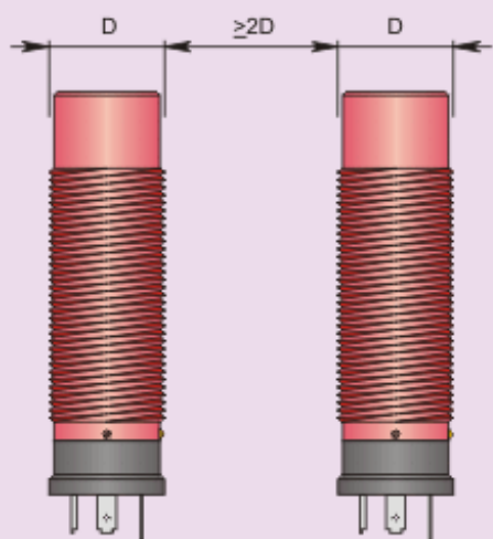
Montaggio affiancato
