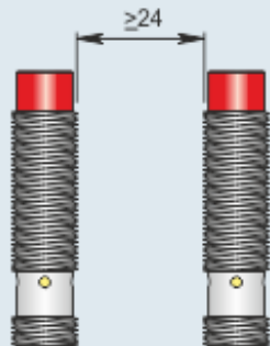
Montaggio affiancato
