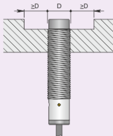
Montaggio sporgente
