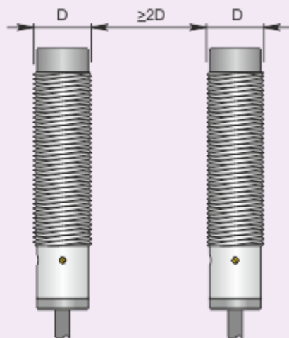
Montaggio affiancato
