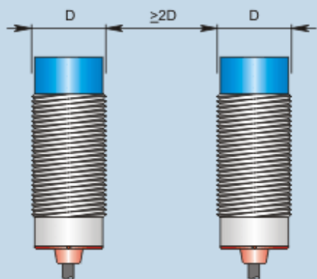
Montaggio affiancato
