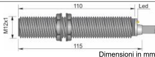
Dimensioni in mm
