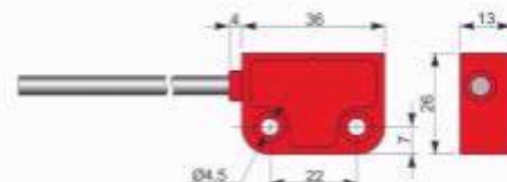
Dimensioni in mm
