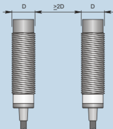
Montaggio affiancato
