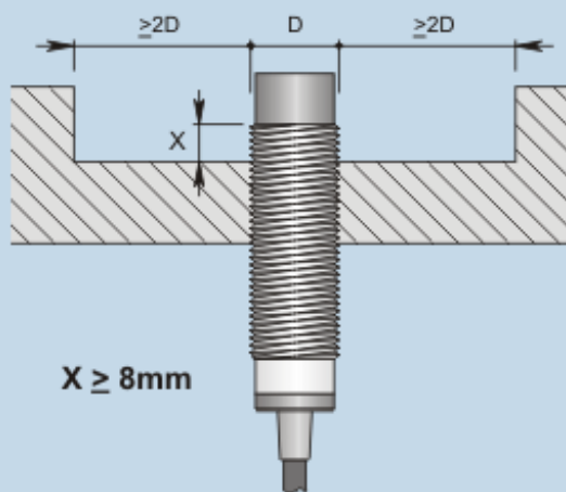
Montaggio sporgente
