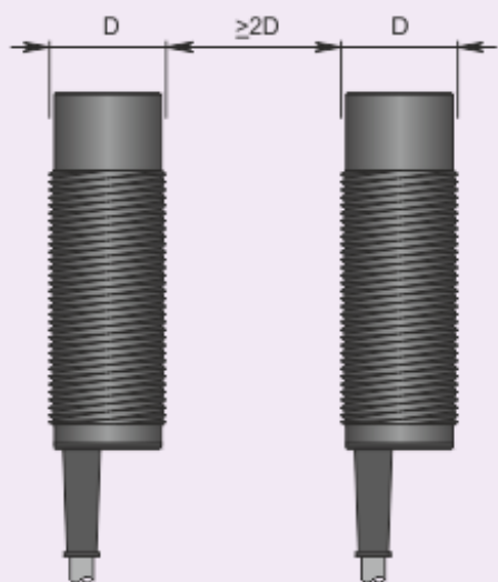
Montaggio affiancato
