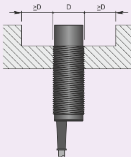
Montaggio sporgente
