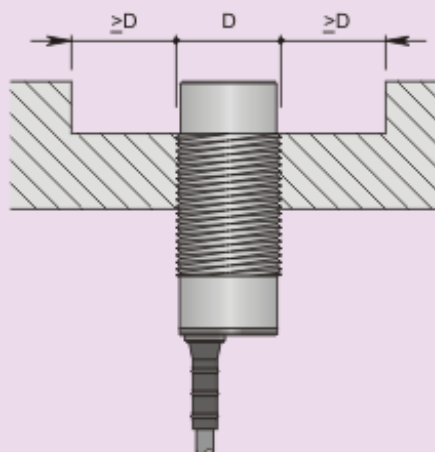
Montaggio sporgente
