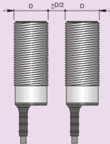
Montaggio affiancato
