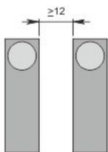
Montaggio affiancato
