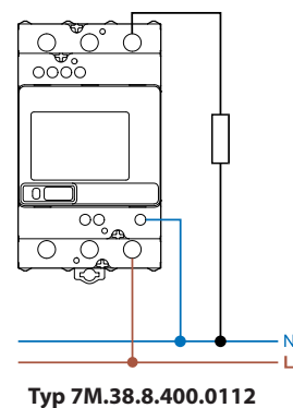
1-fázový systém
