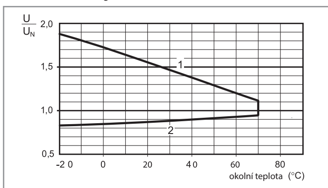
R 62 - pracovní rozsah DC cívky - Z se zhášecím magnetem
