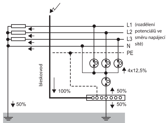
rozdělení bleskového proudu I (10/350 \mu s)
