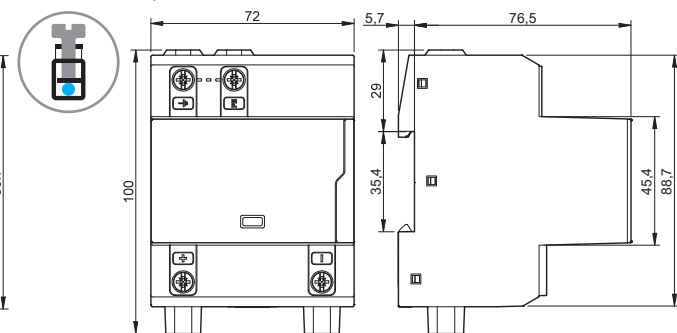
Typ 7P.13.9.500.x006 šroubové svorky
