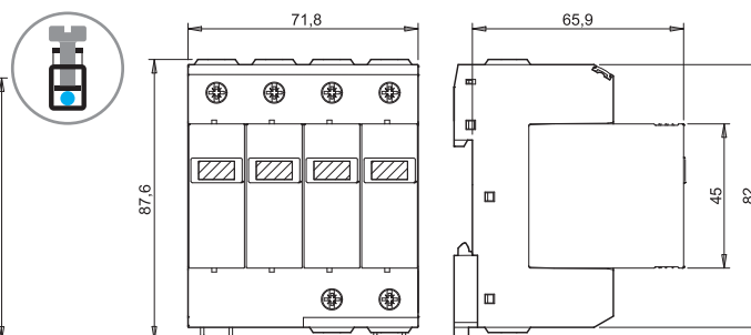
Typ 7P.25/ /7P.45 šroubové svorky
