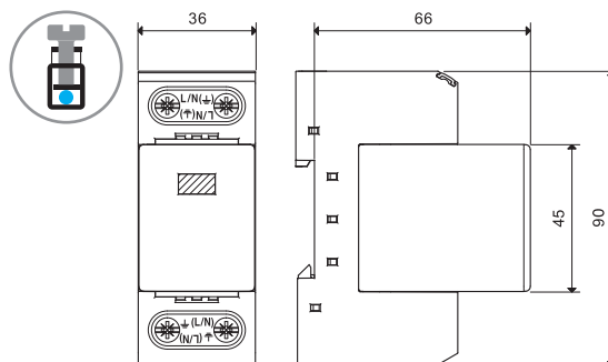
Typ 7P.01 šroubové svorky
