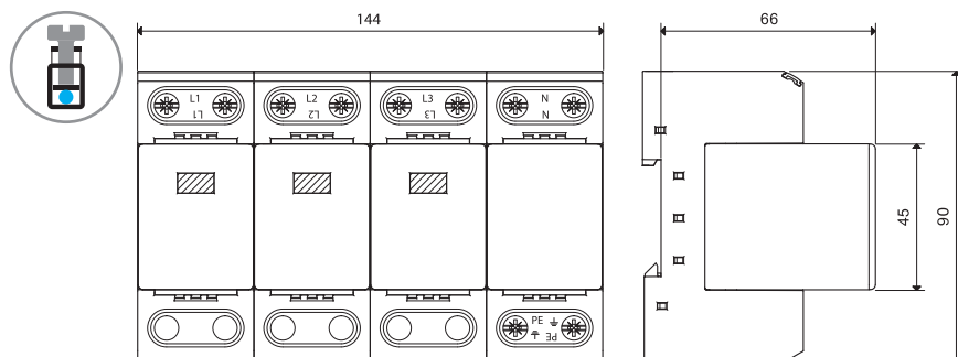
Typ 7P.04 šroubové svorky
