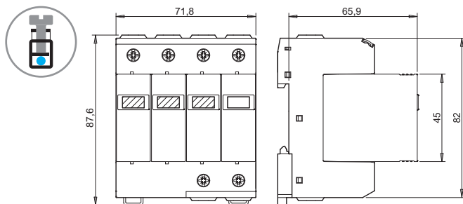
Typ 7P.14 šroubové svorky
