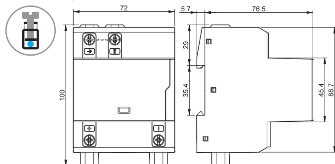
Typ 7P.13.9.000.x006 šroubové svorky
