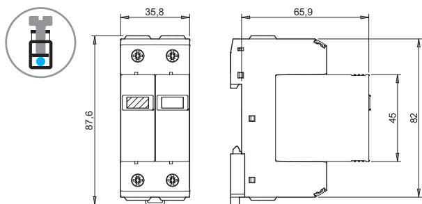
Typ 7P.12 šroubové svorky
