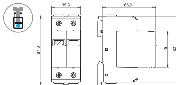
Typ 7P.13 šroubové svorky
