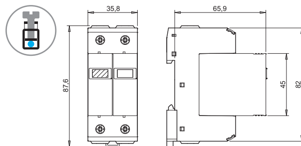
Typ 7P.22 / 7P.27 / 7P.42 šroubové svorky
