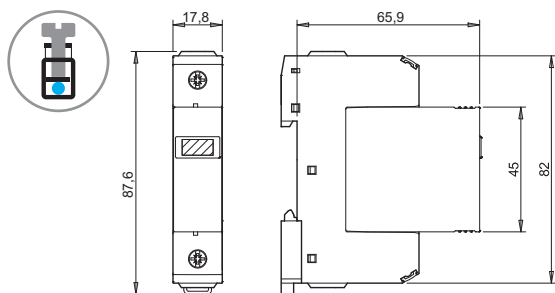
Typ 7P.21 šroubové svorky
