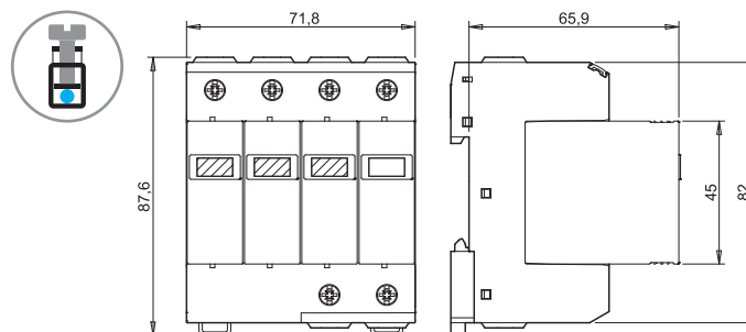
Typ 7P.24/ 7P.44 šroubové svorky
