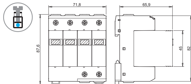
Typ 7P.15 šroubové svorky
