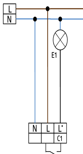
Schéma zapojení
