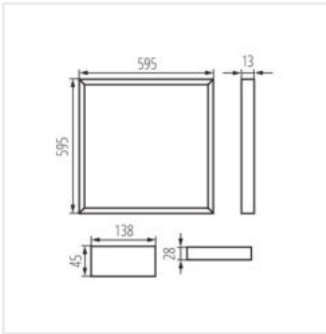
AVAR U 6060 32W-NW
