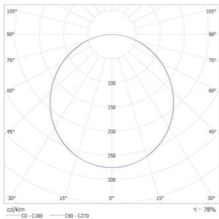
MILED o (kat 31169) BAREV ECO 36W 6060NW / Krzywa rozsyłu światła (biegunowo)
