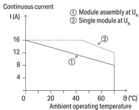
Křivka proudové zatížitelnosti
