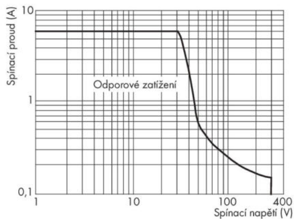
DC křivka mezního zatížení
