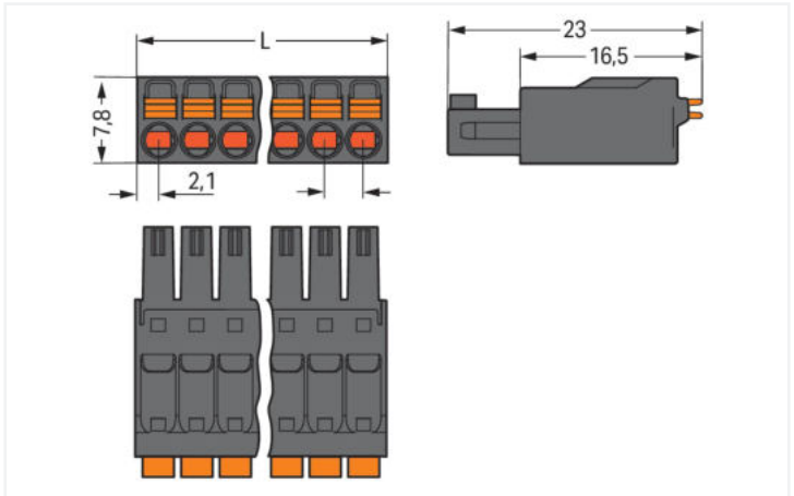
Rozměry v mm L = (počet pólů – 1) × rozteč + 4,2 mm
