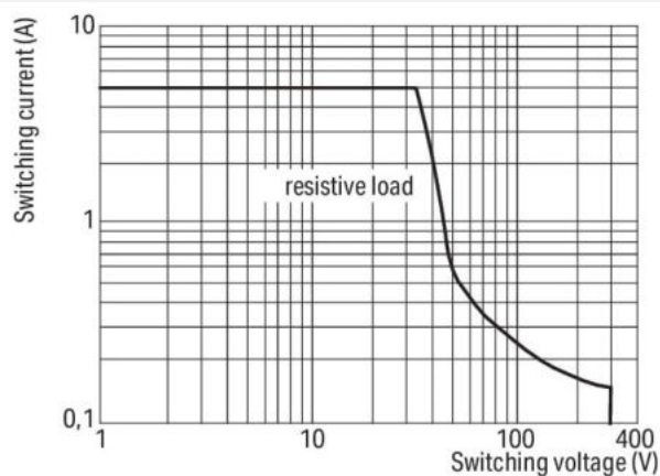
DC křivka mezního zatížení
