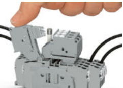
Pojistková svorka s výklopným držákem pojistek Držák pojistky vyklopte do otevřené (aretované) polohy.
