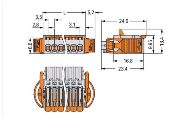
L = (\text{počet pólů} \times \text{rozteč}) + 2,4 \text{ mm}
